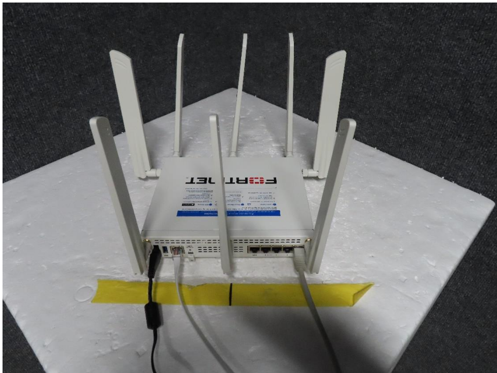
EUT-UNII-2a
